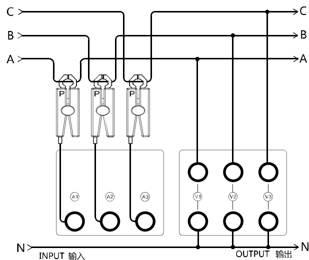
三相四线经 CT 三元测量。
