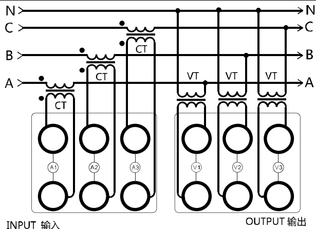
三相四线经 CT-VT 三元测量。
